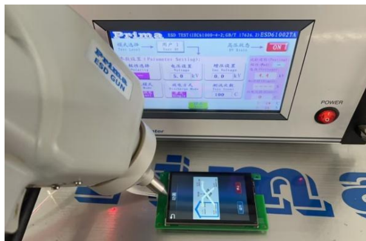
图 4-2 ESD 测试图
