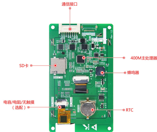
图 1-4 硬件配置图
