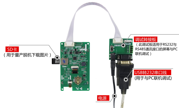
图 1-5 RS232 调试工具图
