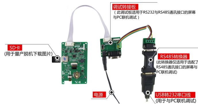
图 1-6 RS485 调试工具图
