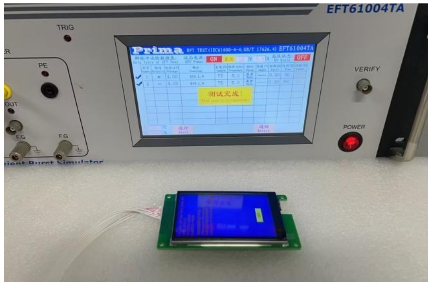
图 4-3 EFT 测试图
