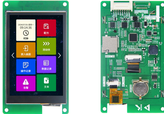
图 1-1 3.5 寸电容触摸参考图
