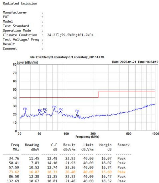
图 4-7 RE 测试垂直方向
