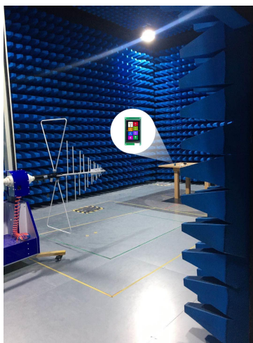
图 4-5 RE 测试图
