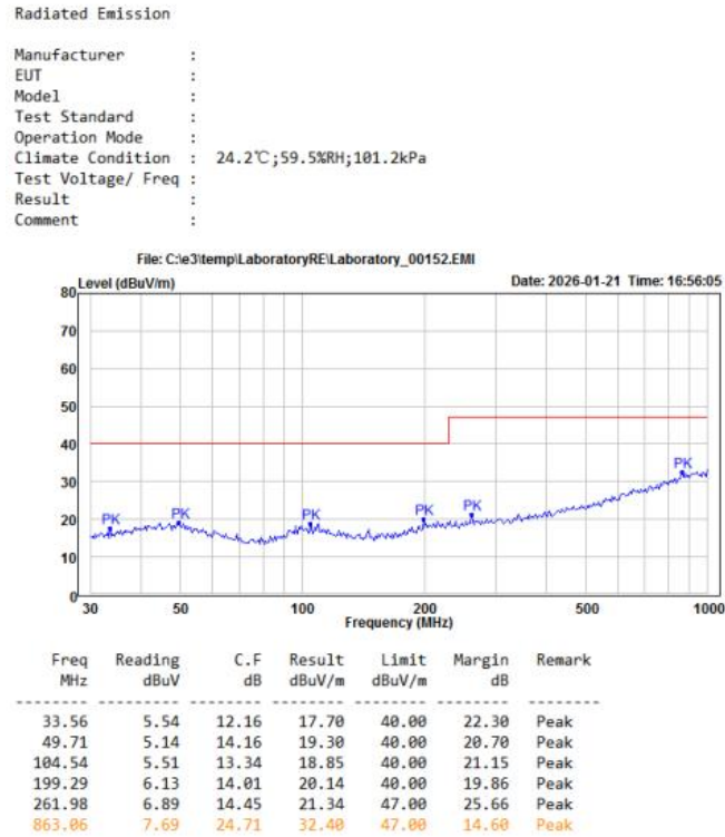
图 4-6 RE 测试水平方向
